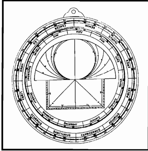
اصطرلاب کا پشت والا حصہ
