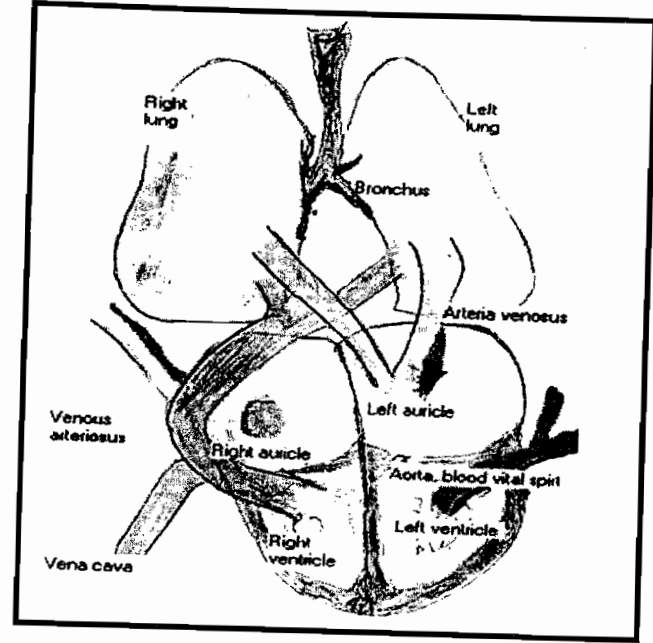
ابن النفیس کی تھیوری آف پلمونری سرکولیشن کی وضاحت
